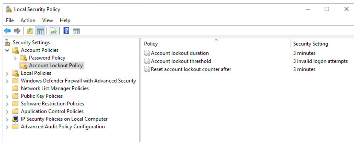
Abbildung 5: Regeln für Kontensperrung
