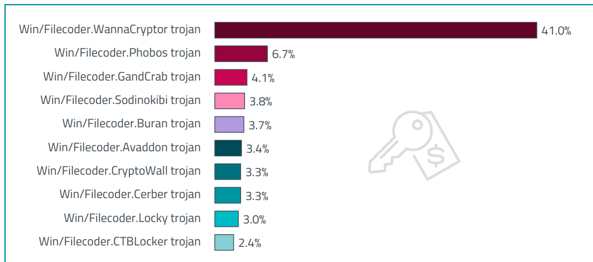
Abbildung 4: Auch vier Jahre nach der ursprünglichen Kampagne im Jahr 2017 ist WannaCryptor eine der am häufigsten beobachteten Ransomware-Familien (Quelle: ESET Threat Report T1, 2021 )
