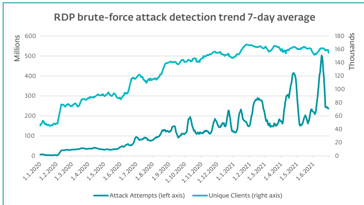
Abbildung 3: Trends der Angriffsversuche auf RDP und Einzel-Clients zwischen Januar 2020 und Juni 2021, gleitendes 7-Tages-Mittel
